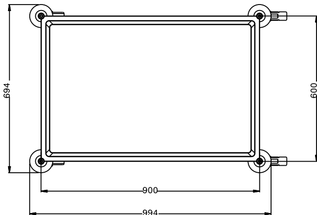
Boven aanzicht
